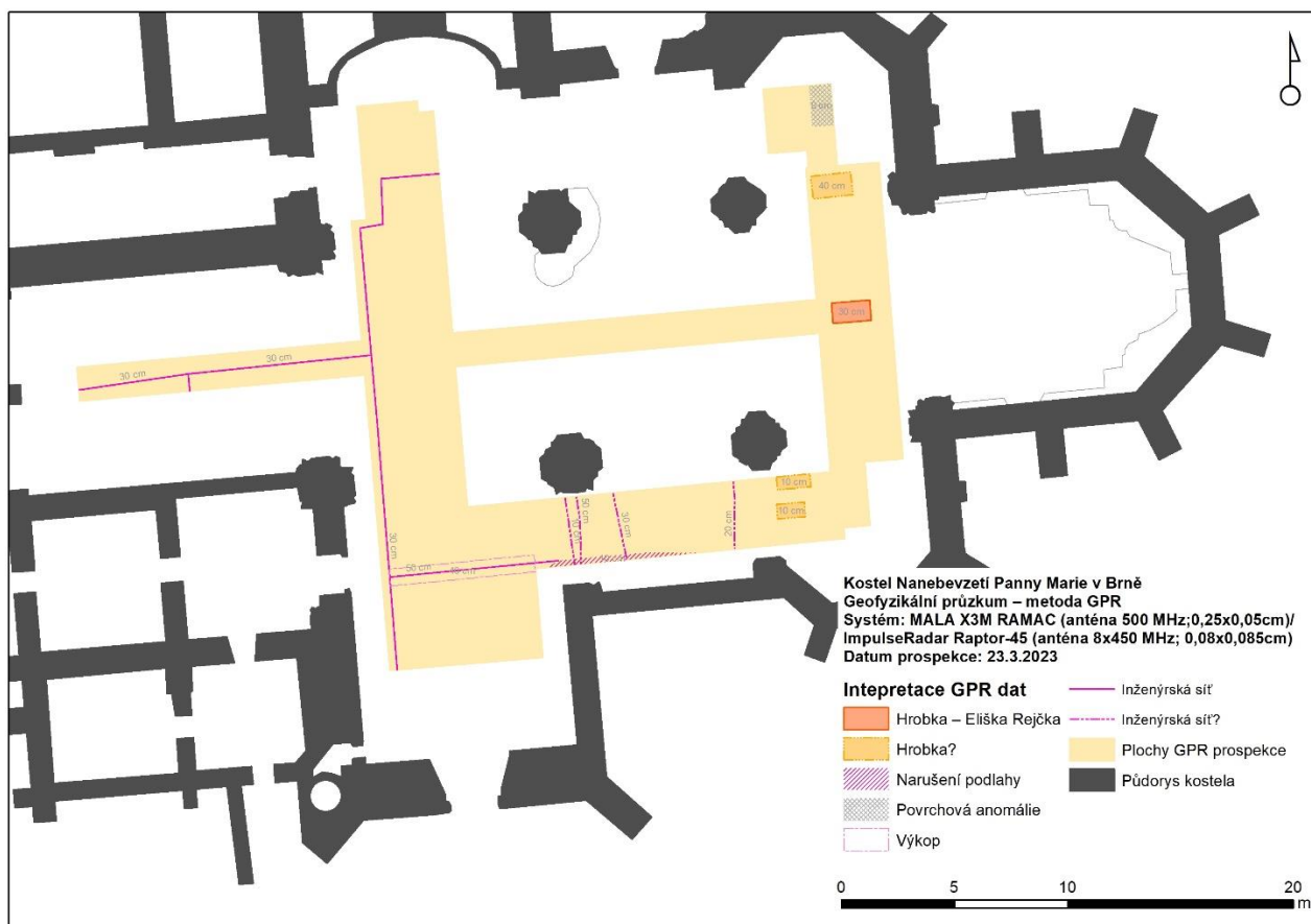
Výsledky geofyzikálního průzkumu v kostele Panny Marie na Starém Brně.
